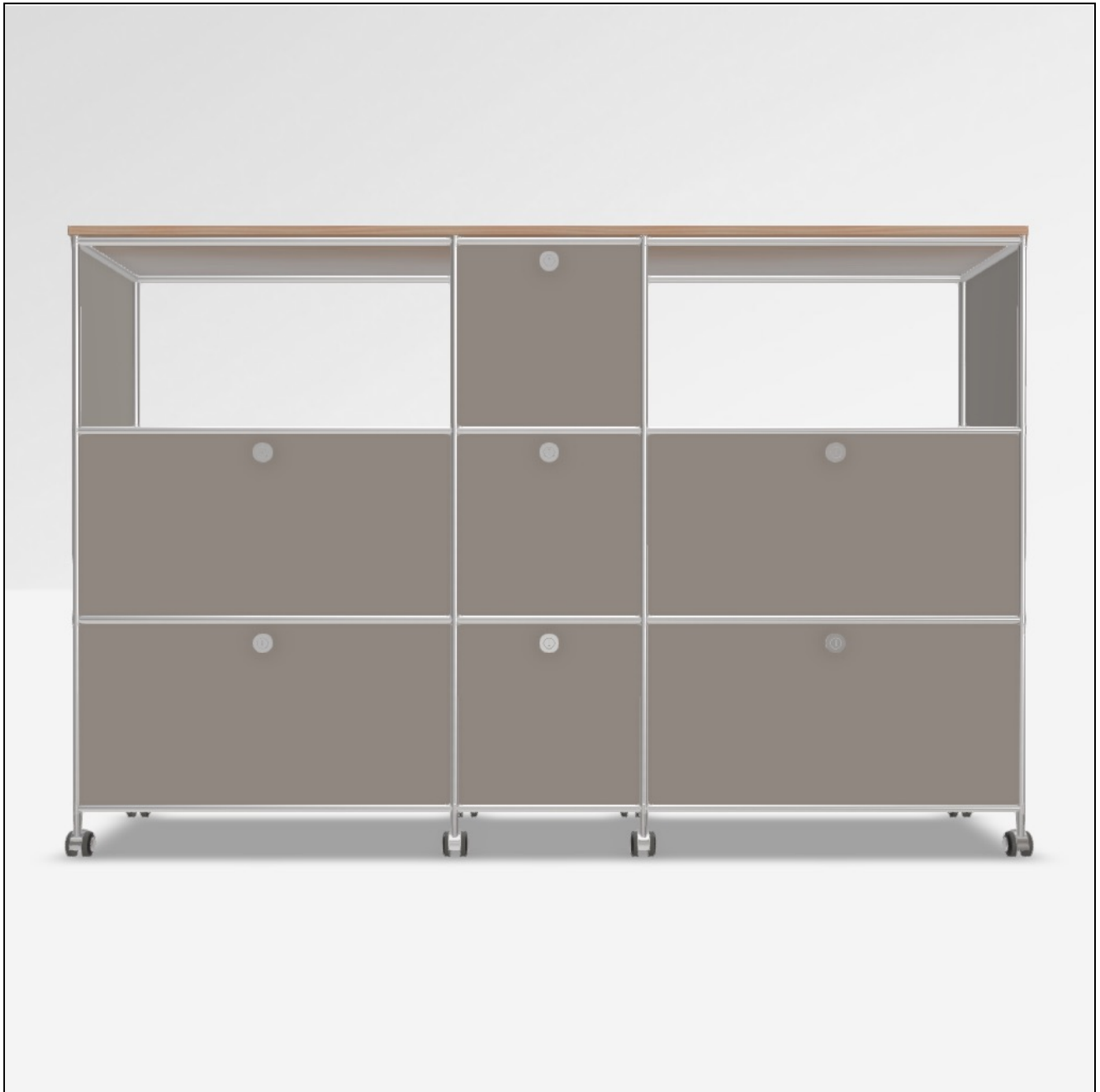
Konfiguration: Personalisiertes Fach, Klappe unten, Personalisiertes Fach # Klappe unten, Klappe unten, Klappe unten # Schublade, Klappe unten, Schublade
